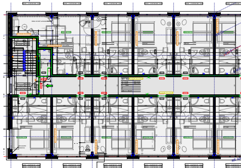
Werkpläne
